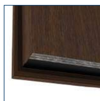
Przylga dolna + uszczelka szczotkowa w skrzydle
